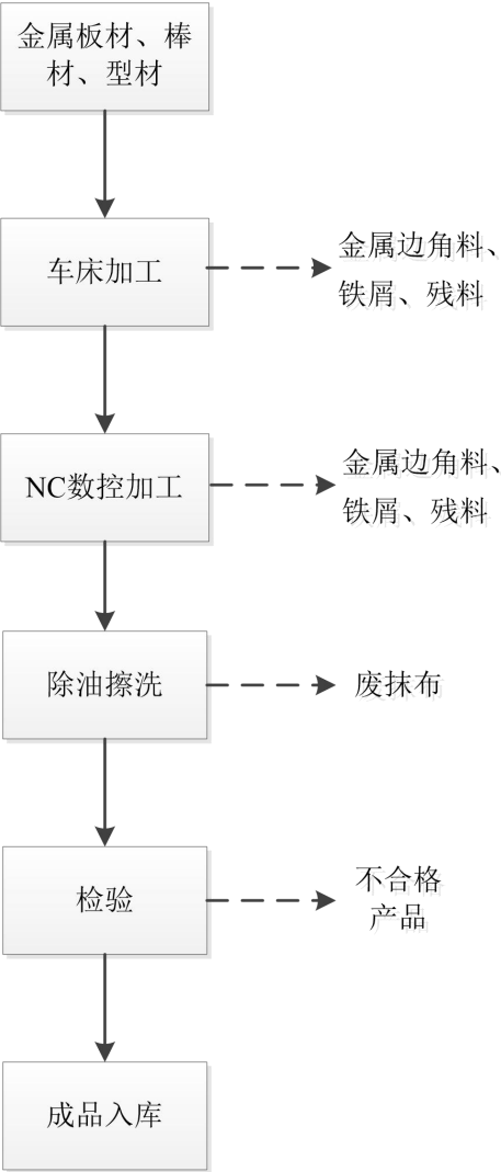
图 2.9-2 机加工产品工艺流程
