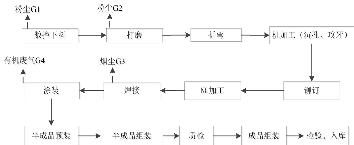
图 2.9-1 工艺流程及产排污环节示意图
