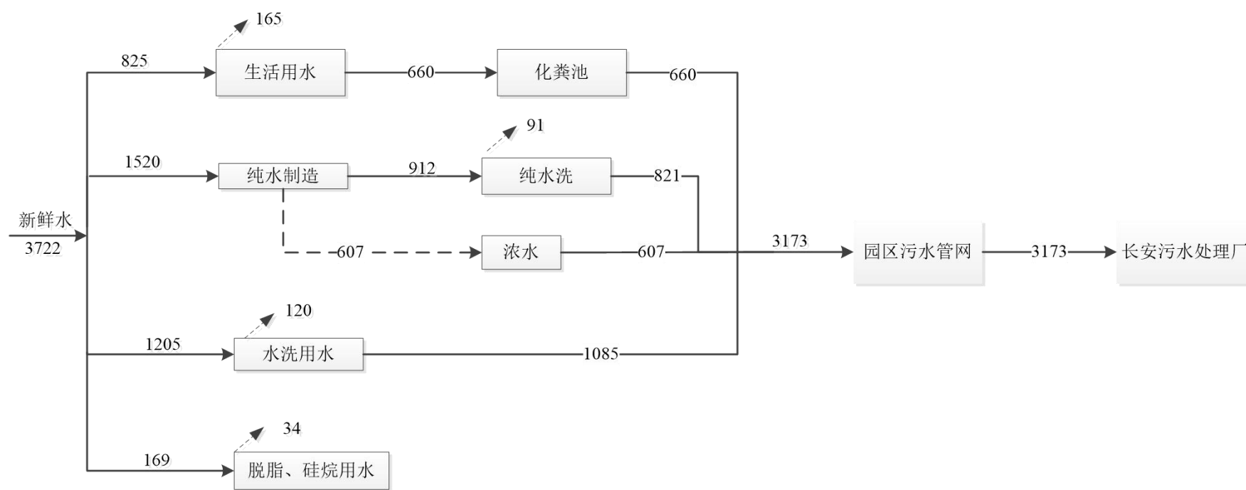
图 2.7-1 水平衡图 (m³/a)
