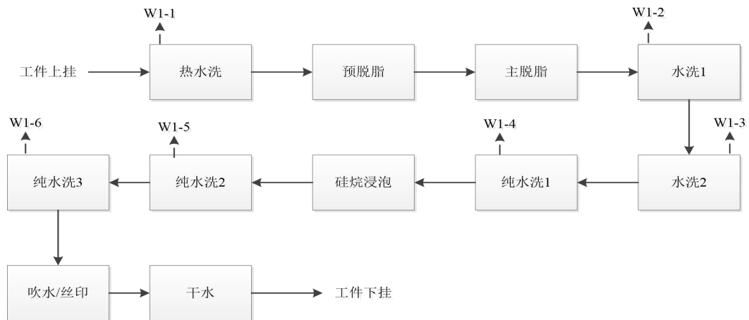
图 2.9-3 喷涂前处理工艺流程
