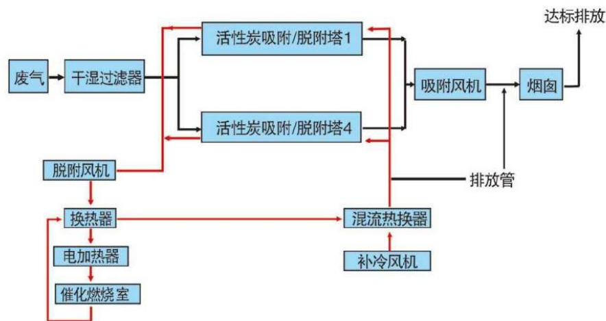
图 4.1-1 活性炭吸附装置+催化燃烧工艺流程
