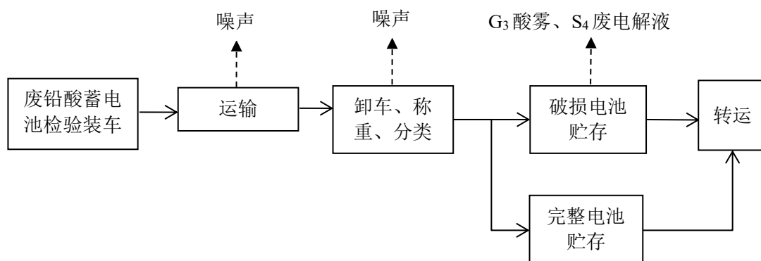
图 2.8-2 废铅酸蓄电池收集贮存流程及产污环节图
