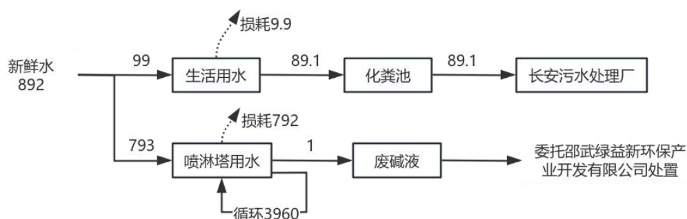
图 2.7-1 项目及全厂水平衡图 t/a
