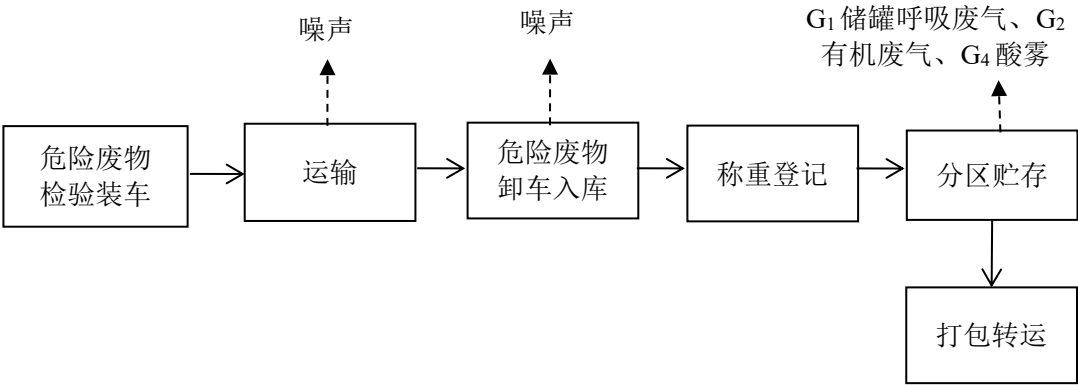
图 2.8-1 危险废物收集贮存流程及产污环节图
