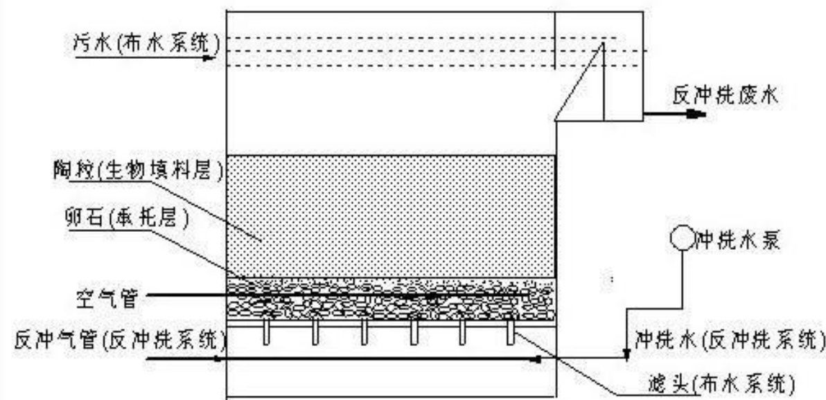
图4.4.5-4 生物滤池结构示意图
