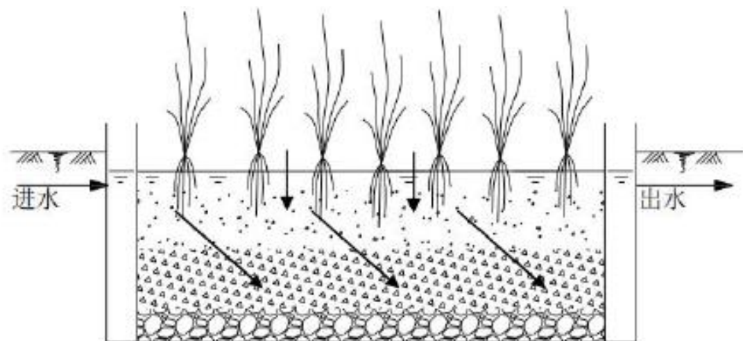
图4.4.5-7 水平潜流人工湿地示意图
