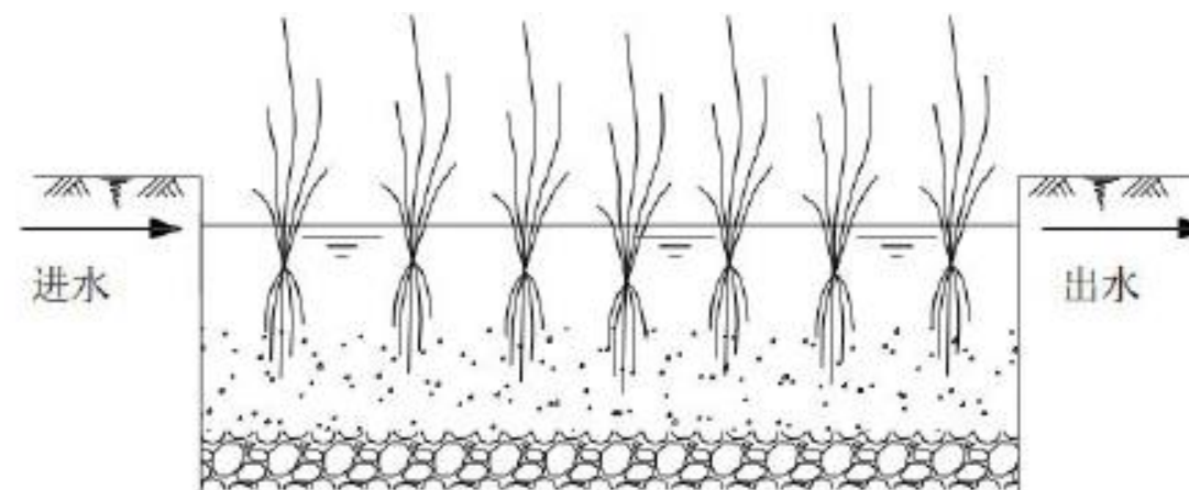
图4.4.5-6 表面流人工湿地示意图
