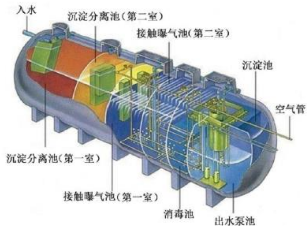
图4.4.6-5 净化槽构造示意图
