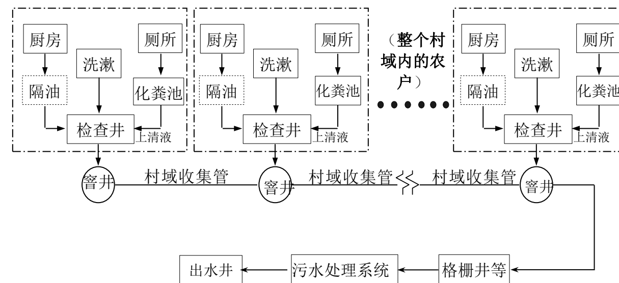
图4.4.4-2 按片区集中收集处理模式
