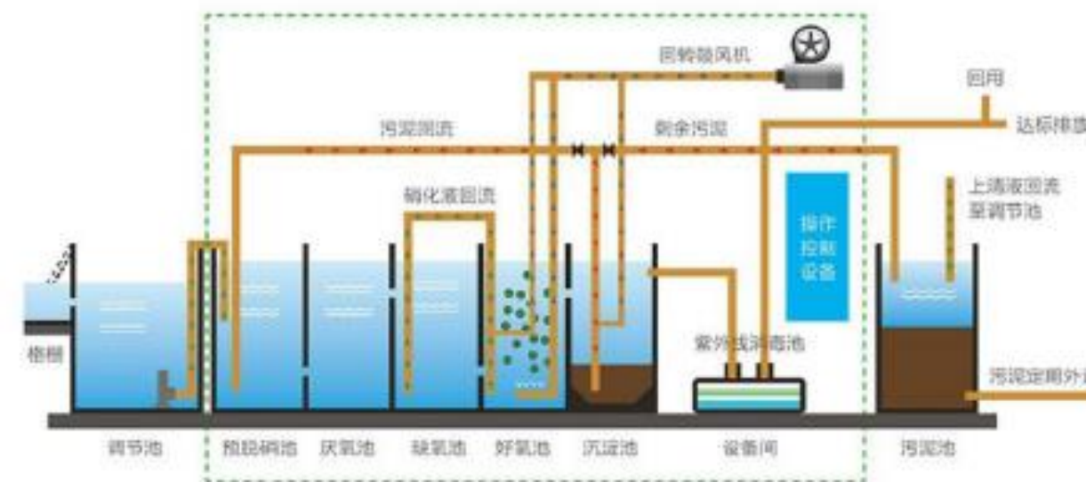
图4.4.6-6 A3/O 移动床生物膜反应器污水处理装置构造图
