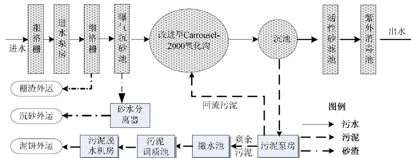
图4.1-1 琅岐污水处理厂处理工艺流程图
