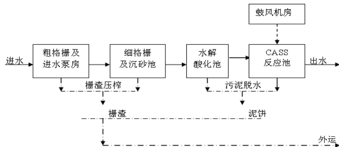
图4.1-5 长安污水处理厂处理工艺流程图
