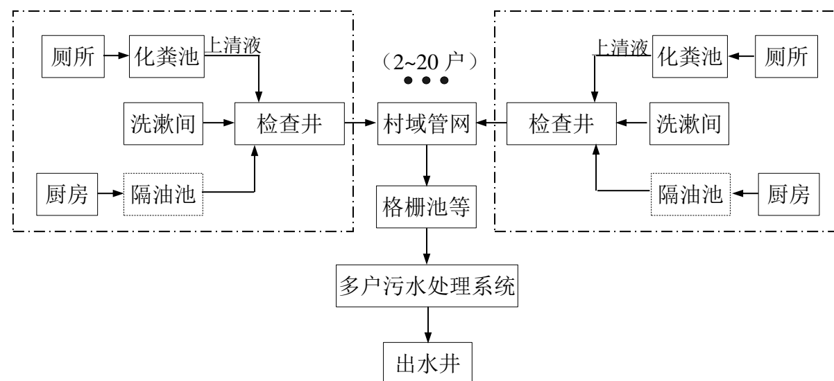
图4.4.4-4 多户式污水收集处理模式
