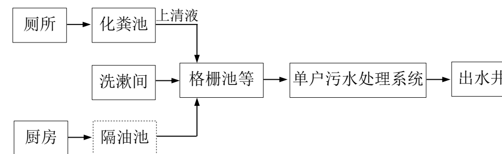
图4.4.4-3 单户式污水收集处理模式
