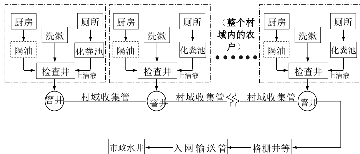
图4.4.4-1 生活污水纳厂处理模式
