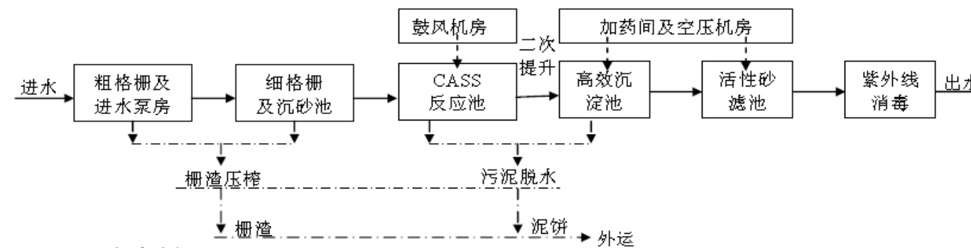
图4.1-6 长安污水处理厂提标改造处理工艺流程图
