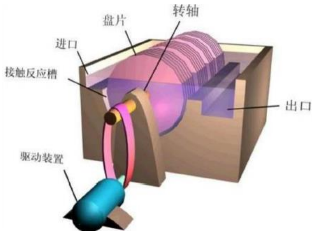
图4.4.5-5 生物转盘结构示意图
