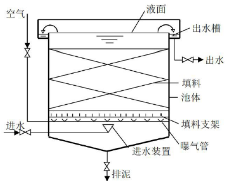
图4.4.5-3 厌氧生物膜池结构示意图
