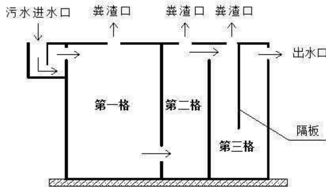
图4.4.5-1 三格化粪池典型结构
