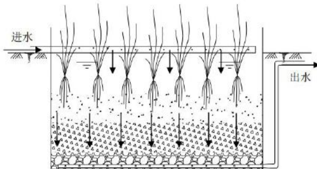
图4.4.5-8 垂直潜流人工湿地示意图
