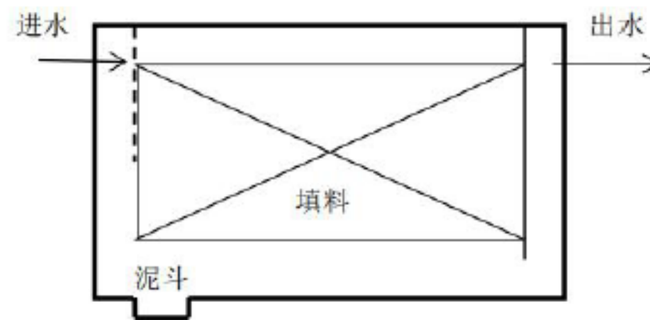
图4.4.5-2 厌氧生物膜池结构示意图
