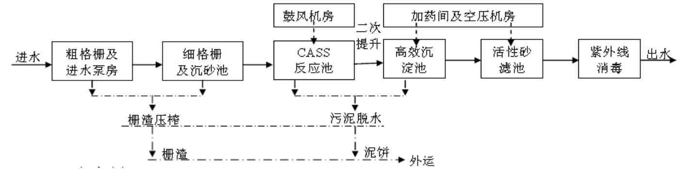
图4.1-6 长安污水处理厂提标改造处理工艺流程图
