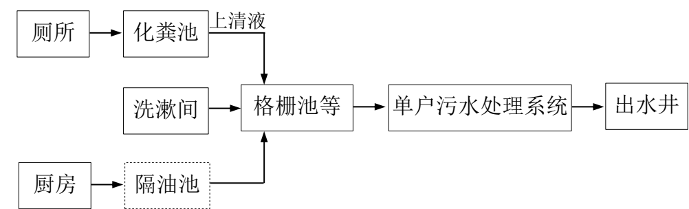
图4.4.4-3 单户式污水收集处理模式
