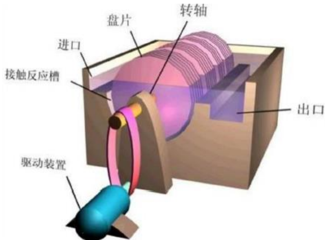
图4.4.5-5 生物转盘结构示意图
