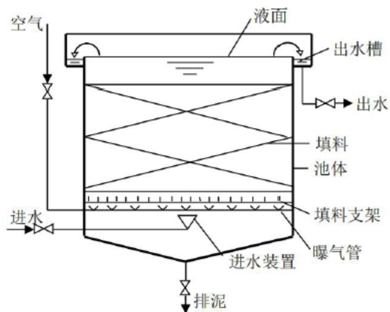
图4.4.5-3 厌氧生物膜池结构示意图
